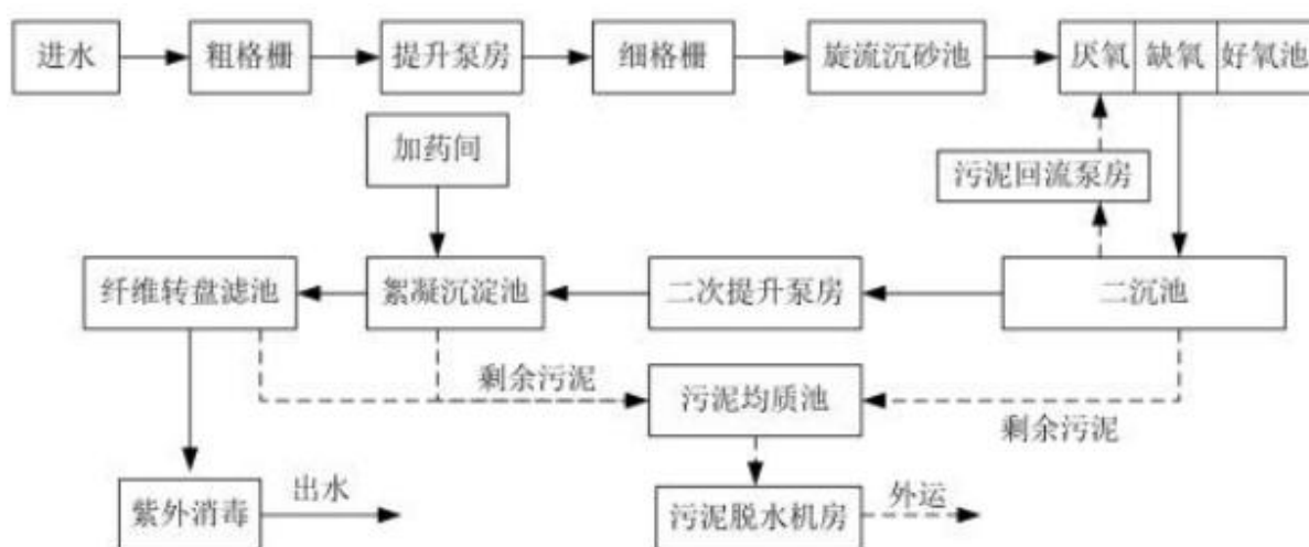
图 1 污水厂原有工艺流程
