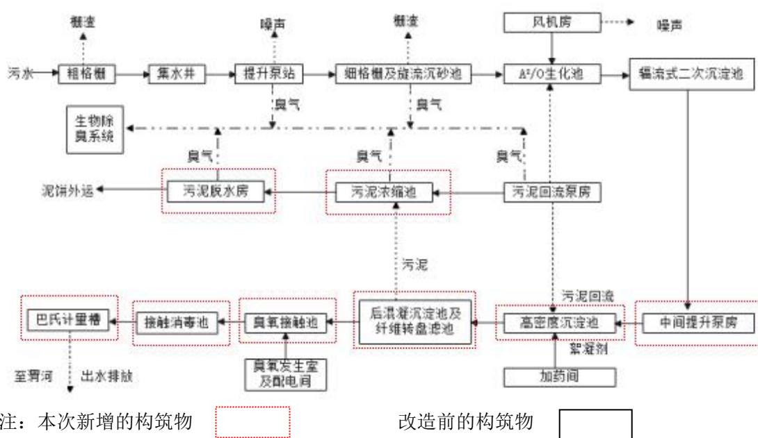
图3 工程运营期工艺流程及产污环节图
