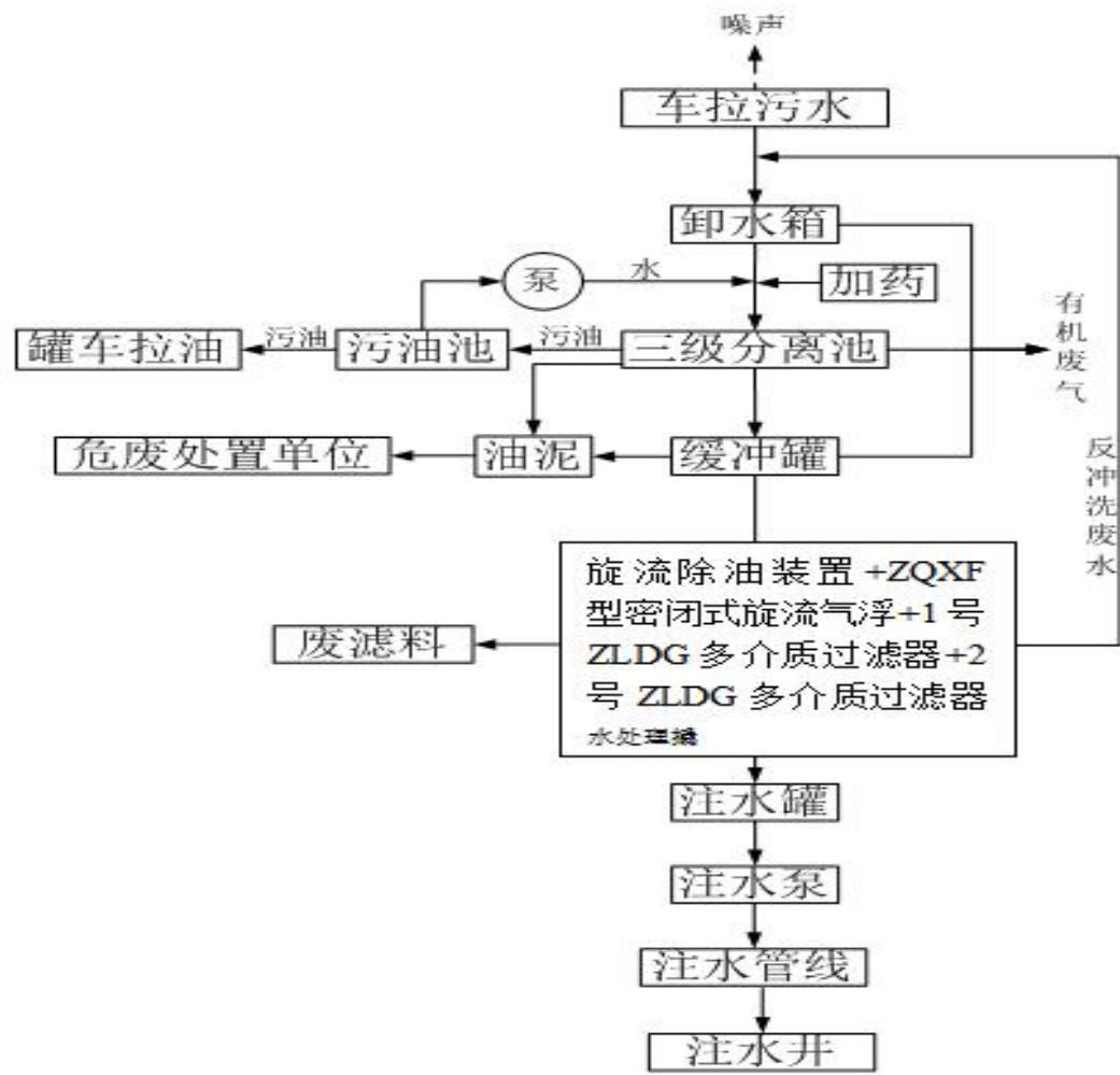
图 2-1 项目运营期生产工艺及产污环节图
