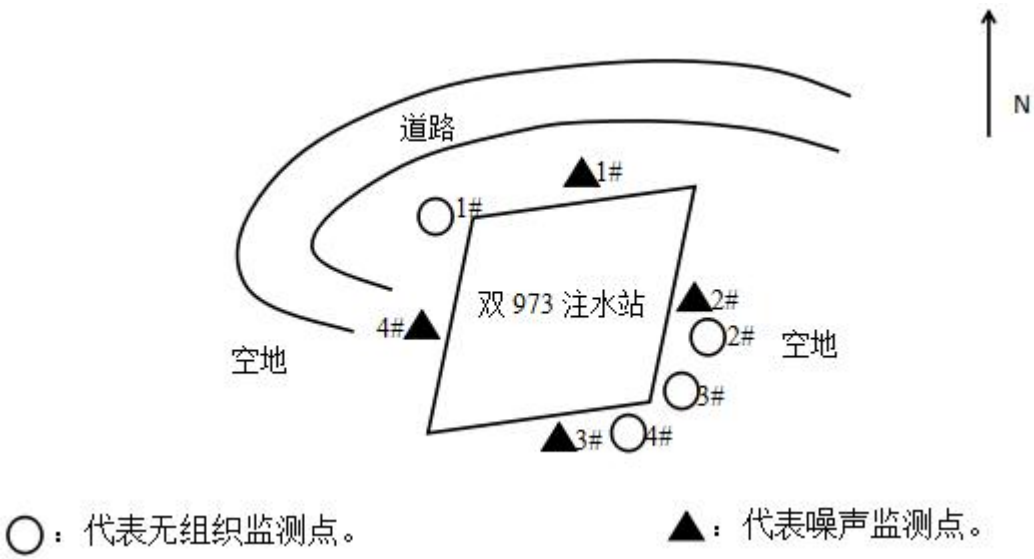
图 5-1 验收监测点位布设示意图
