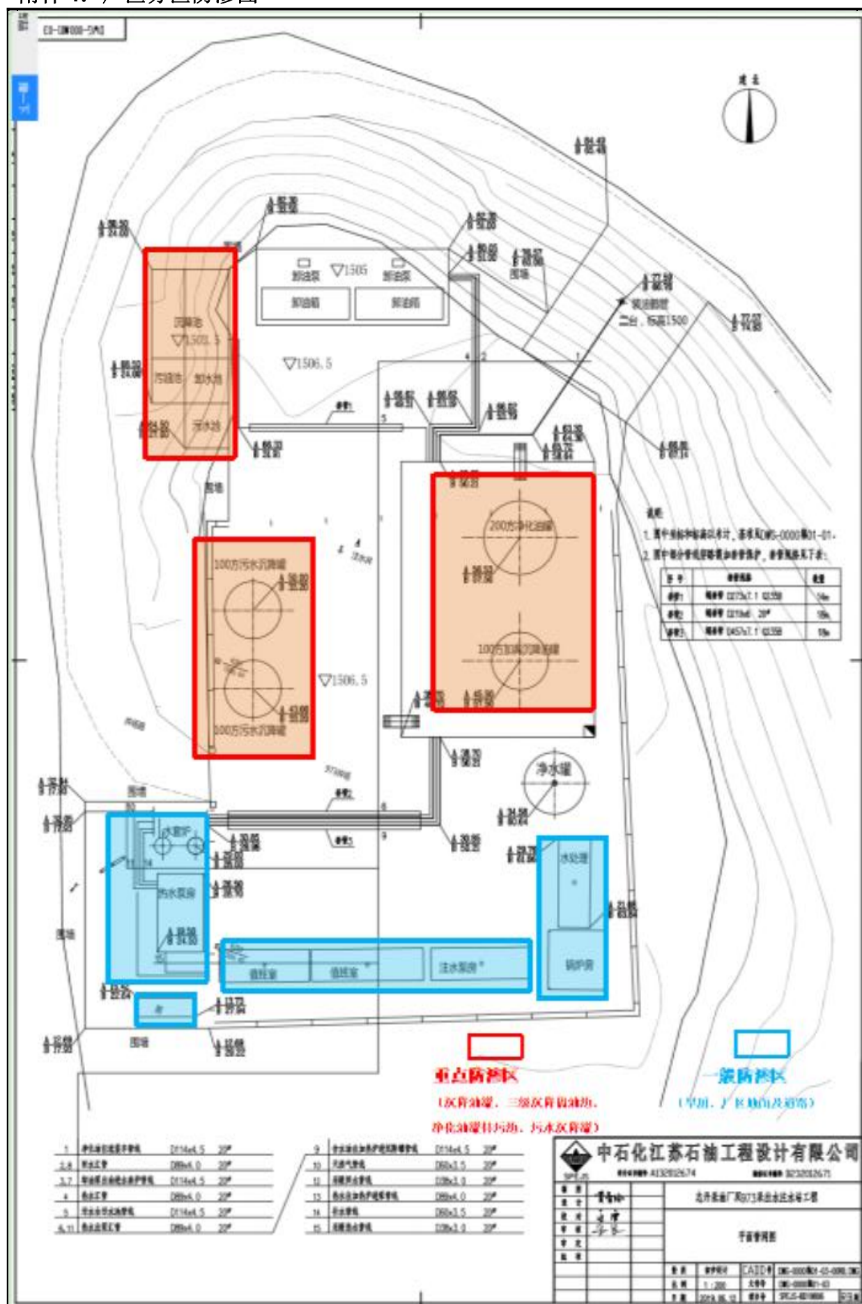
附件 4：厂区分区防渗图
