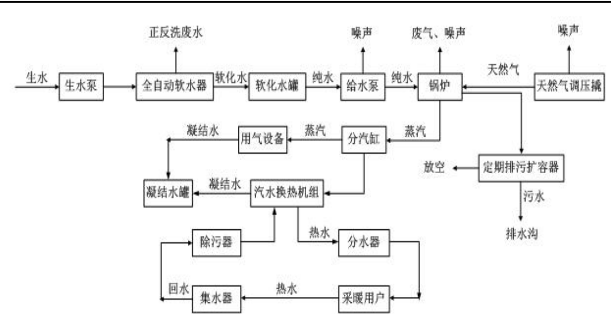
图 2-1 项目锅炉煤改气工艺流程和产污环节图
