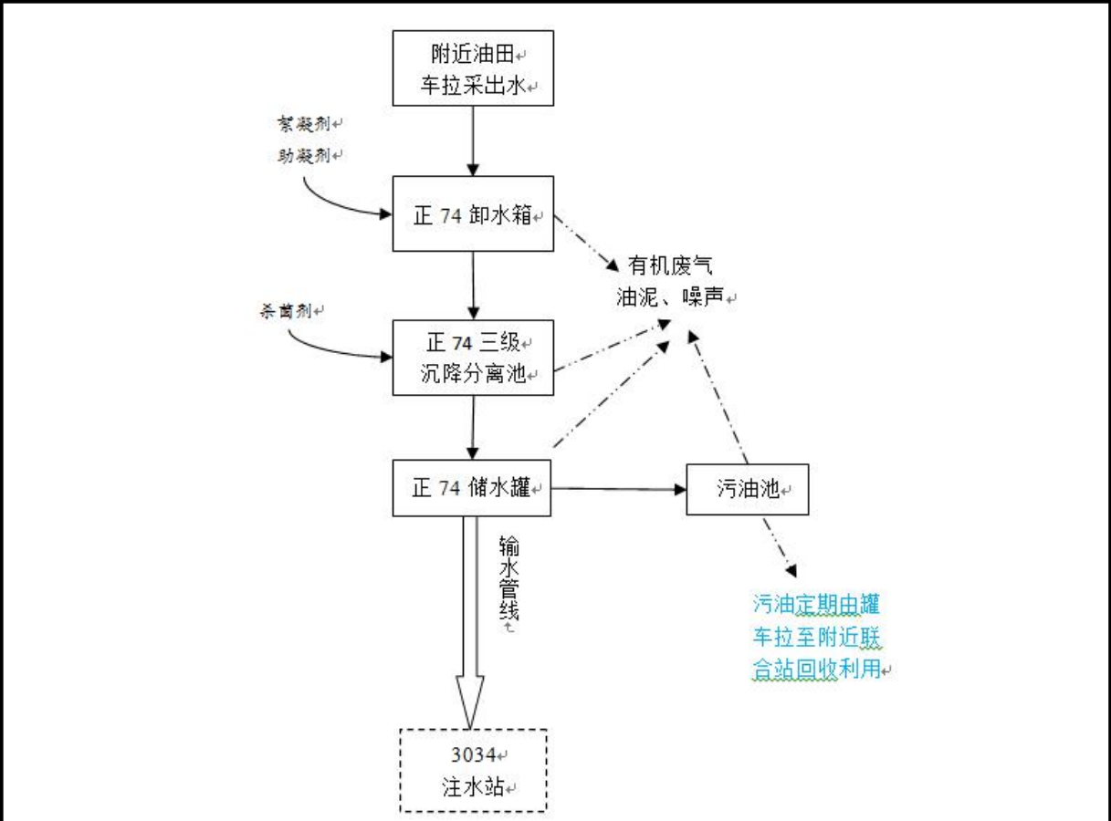
图 2-1 项目运营期生产工艺及产污环节图
