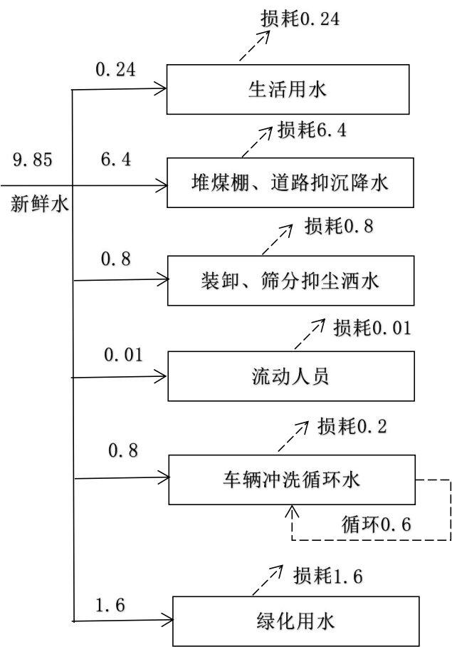
图2-4 项目水平衡图
