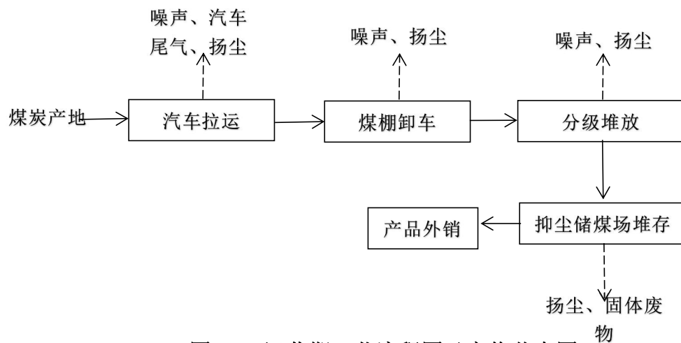
图 2-6 运营期工艺流程图及产物节点图
