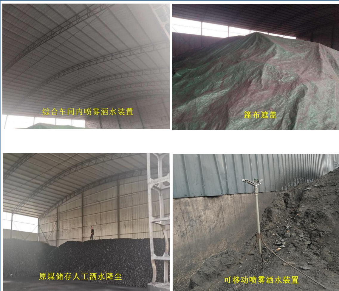
图3-1 废气治理措施图
